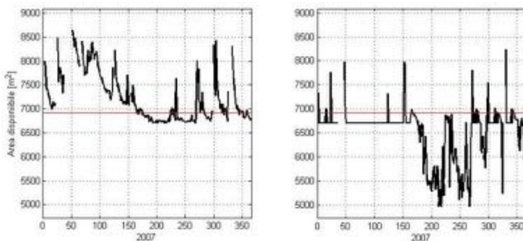
Figura A4.8 - Serie storica di habitat disponibile (espresso in m 2 ) per l'anno 2007 in assenza (grafico di sinistra) e a valle (grafico di destra) della derivazione in esame, con indicata la soglia di riferimento (6918 m 2 , linea continua rossa) definita per la specie barbo sp. – adulto e corrispondente ad una portata Q355 = 0.83 m 3 s -1 . Nella figura non vengono riportati i valori di habitat disponibile relativi a portate maggiori di 4.4 m 3 s -1 in quanto al di fuori dell'intervallo di portate considerato.
