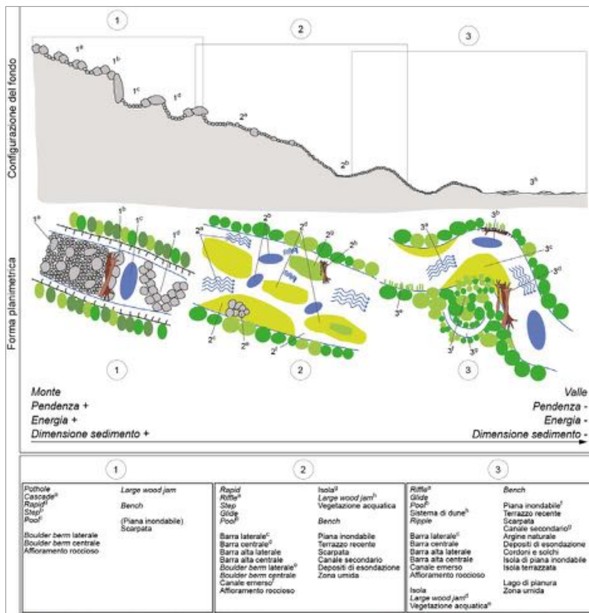
Figura 1.2 - Schema della successione di unità morfologiche lungo un corso d'acqua, da monte a valle, al variare delle condizioni al contorno.
