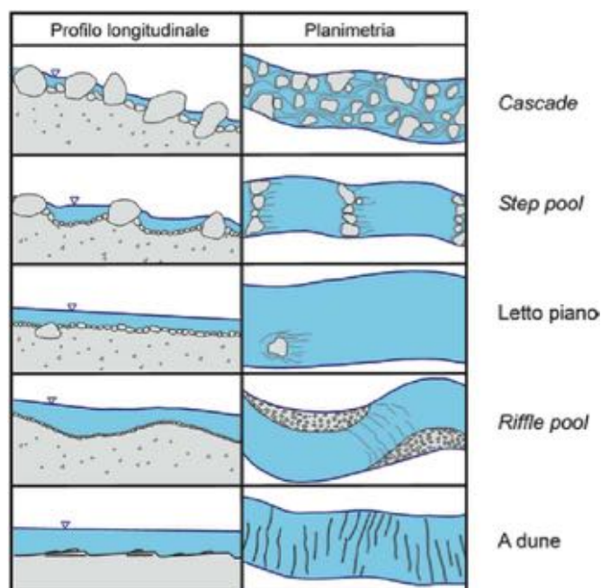
Figura 1.3 - Morfologie di alvei alluvionali a scala di tratto (modificato da Montgomery & Buffington, 1997 ).
