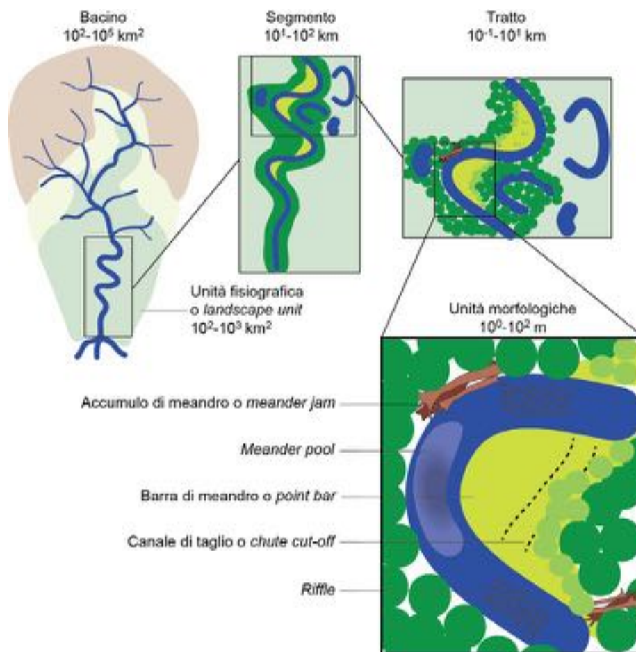
Figura 1.1 - Estratto dell'approccio gerarchico dalla scala del bacino fino alla scala delle unità morfologiche (in basso sono riportate come esempio alcune unità morfologiche).
