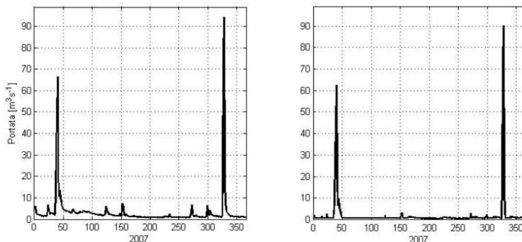
Figura A4.7 - Serie storica di portate medie giornaliere per l'anno 2007 in assenza (grafico di sinistra) e a valle (grafico di destra) della derivazione in esame per il F. Taro a piane di Carniglia.
