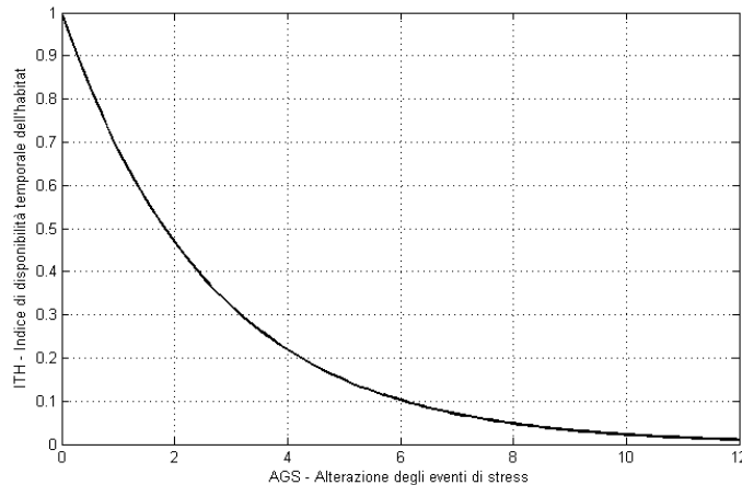
Figura A4.6 - Rappresentazione della funzione di valore per il calcolo dell'indice ITH (indice di disponibilità temporale dell'habitat) basato sull'indicatore AGS (alterazione dei giorni di stress).
