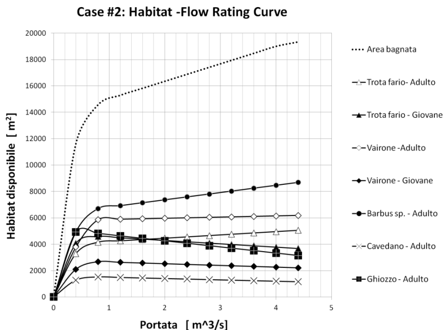
Figura A4.3 - Relazione habitat-portata determinata con la metodologia MesoHABSIM per il caso del F. Taro a Piane di Carniglia (Parma). L'habitat disponibile è quantificato per differenti specie e stadi vitali della comunità ittica locale e viene espresso in m 2 in funzione della portata defluente.
