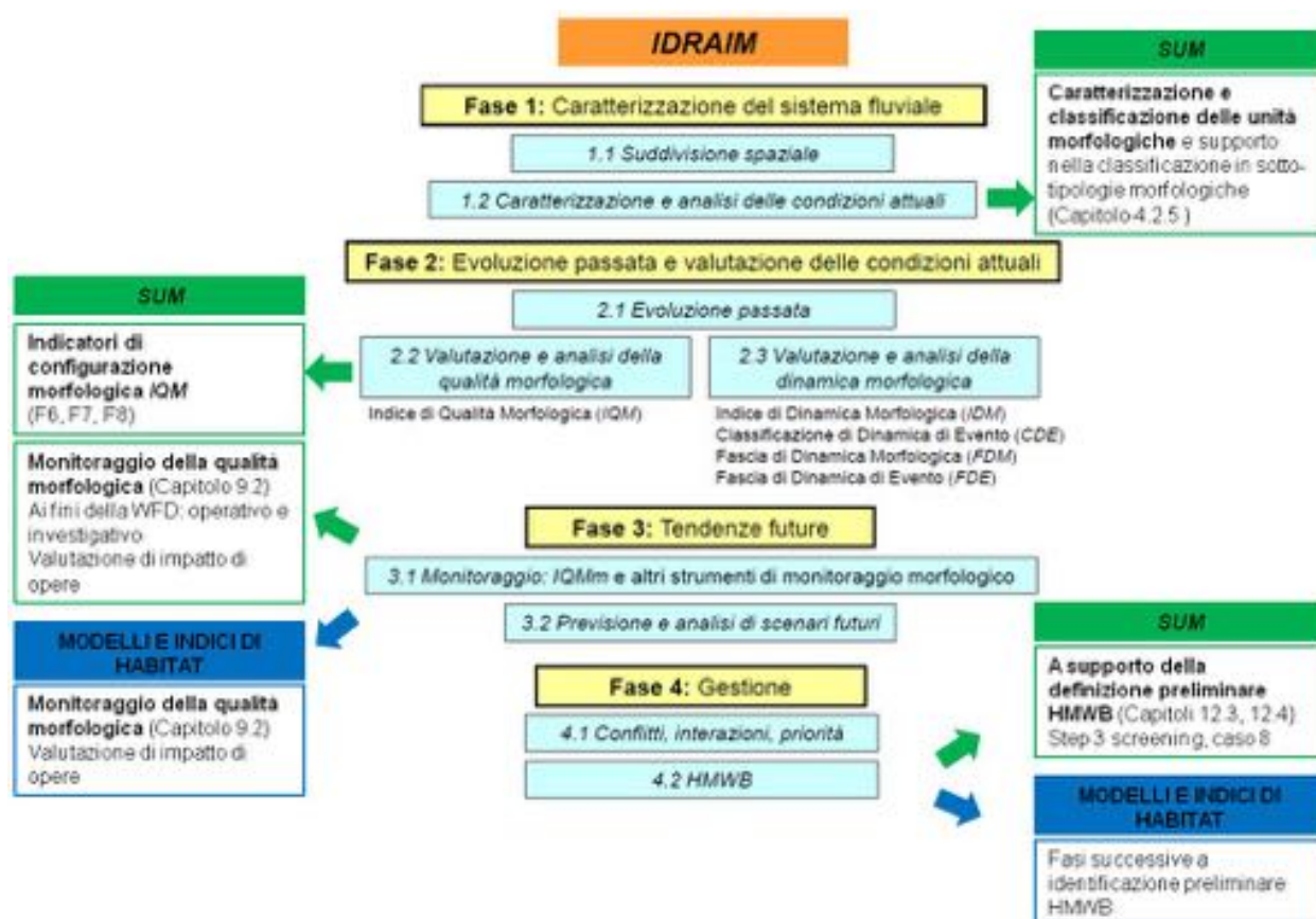
Figura 3.1 - Schema di interazione tra il SUM , i modelli e indici di habitat e la struttura generale del sistema IDRAIM . Modificato da Rinaldi et al. (2014) .
