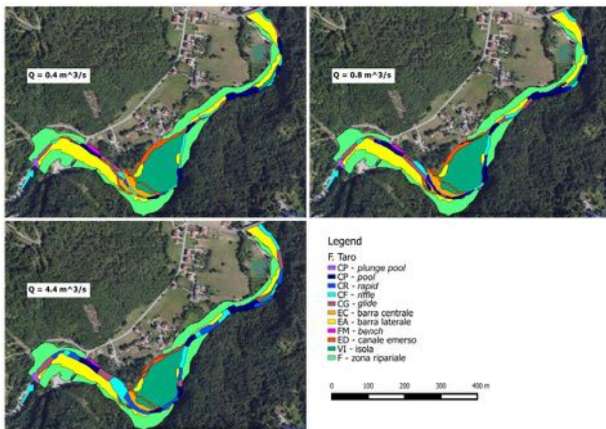
Figura A4.1 - Distribuzione spaziale delle unità morfologiche (unità sommerse e unità emerse) per il caso del Fiume Taro a Piane di Carniglia (Parma) per 3 differenti condizioni di deflusso ( 0.4 \text{ m}^3/\text{s} , 0.8 \text{ m}^3/\text{s} , 4.4 \text{ m}^3/\text{s} ).
