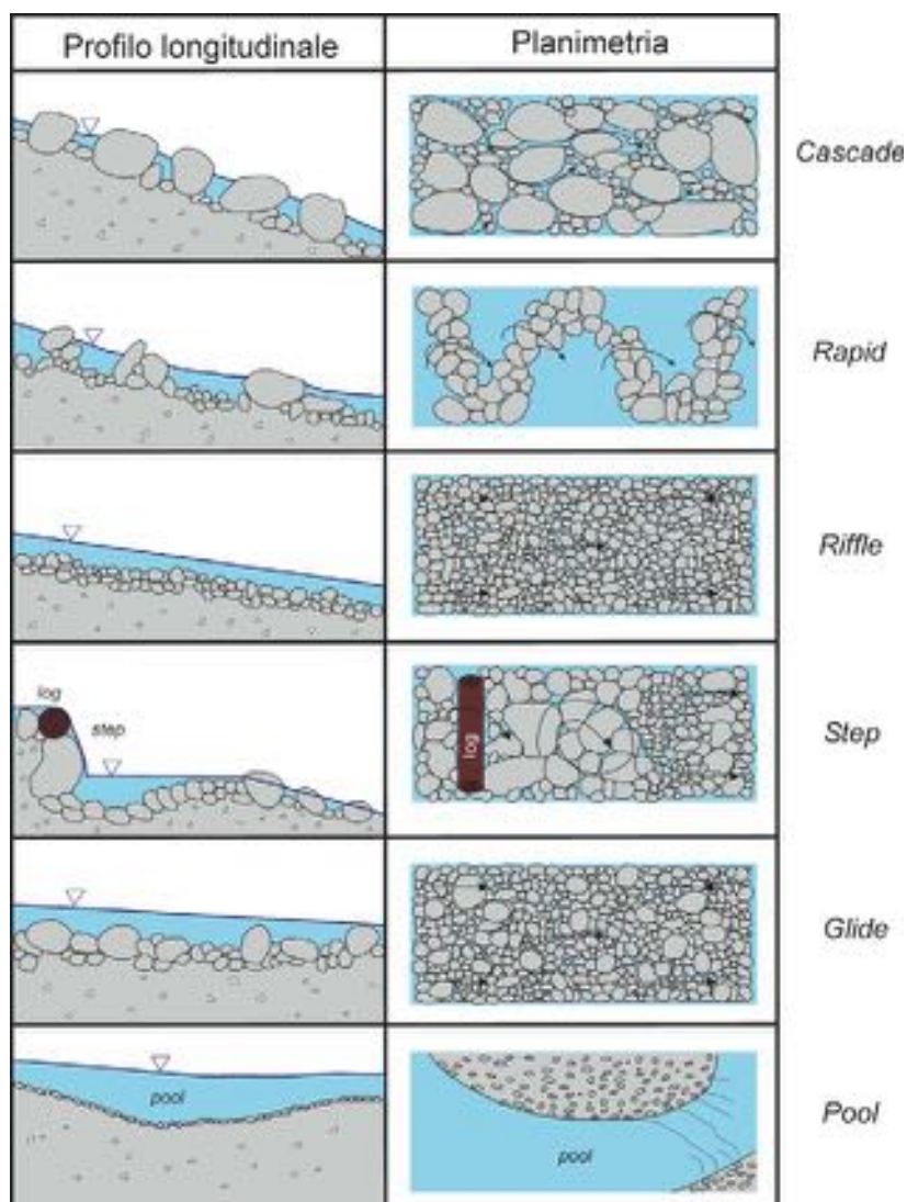
Figura 7.1 - Principali unità di canale in alvei alluvionali a pendenza elevata (modificato da Halwas & Church, 2002 ).
