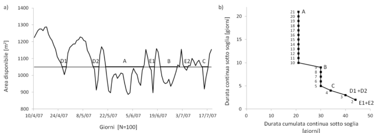
Figura A4.4 - Esempio di calcolo della curva di durata continua sotto-soglia (curva CDS o UCUT). Il calcolo viene eseguito per l'intero intervallo di durate sotto soglia (in Figura: tra 2 – evento E – e 21 giorni – evento A).
