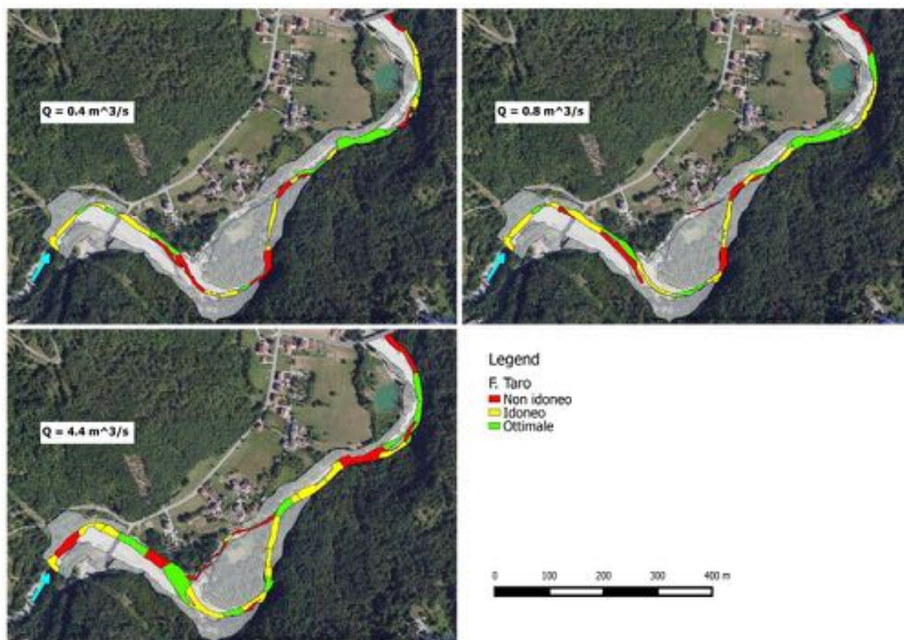
Figura A4.2 - Valutazione in termini di idoneità d'habitat delle unità di canale per il caso del Fiume Taro a Pian di Carniglia (Parma) per 3 differenti condizioni di deflusso ( 0.4 \text{ m}^3/\text{s} , 0.8 \text{ m}^3/\text{s} , 4.4 \text{ m}^3/\text{s} ). Nell'esempio riportato l'habitat viene valutato per il barbo ( Barbus sp., stadio vitale adulto) e classificato secondo 3 categorie: idoneo, non idoneo e ottimale.
