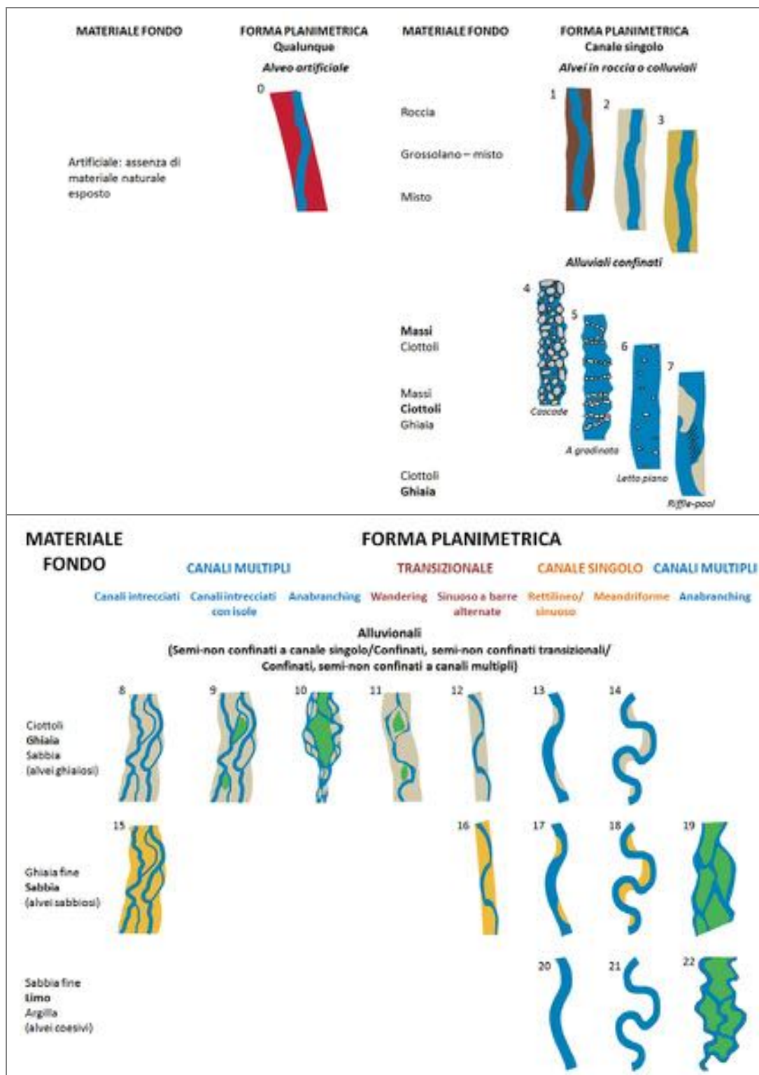
Figura 1.4 - Classificazione estesa delle tipologie morfologiche dei corsi d'acqua ( Extended River Typology ; modificato da Rinaldi et al., 2015 ). Alvei artificiali. (0) A fondo artificiale. Alvei confinati a canale singolo. (1) In roccia; (2) colluviale a sedimenti grossolani - misti; (3) colluviale a sedimenti misti; (4) cascade ; (5) a gradinata; (6) letto piano; (7) riffle-pool . Alvei alluvionali semiconfinati o non confinati a canale singolo, confinati/semi-non confinati transizionali o a canali multipli. (8) A canali intrecciati ghiaioso; (9) a canali intrecciati con isole; (10) anabranching ghiaioso (equiv. ai tipi 3, 5 o 6 secondo Nanson & Knighton (1996) ); (11) wandering ; (12) sinuoso a barre alternate ghiaioso; (13) rettilineo-sinuoso ghiaioso; (14) meandriforme ghiaioso; (15) a canali intrecciati sabbioso; (16) sinuoso a barre alternate sabbioso; (17) rettilineo-sinuoso sabbioso; (18) meandriforme sabbioso; (19) anabranching sabbioso (equiv. ai tipi 2 o 4 secondo Nanson & Knighton (1996) ); (20) rettilineo-sinuoso limoso; (21) meandriforme limoso; (22) anastomizzato (equiv. al tipo 1 secondo Nanson & Knighton (1996) ).
