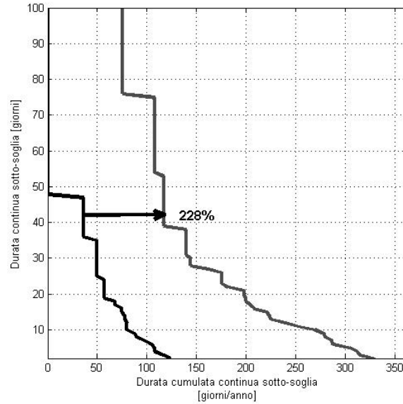
Figura A4.5 - Esempio di calcolo dell'alterazione media della durata degli eventi di stress (eventi di habitat disponibile sotto-soglia) per la specie barbo ( Barbus sp.) per il F. Taro a Piane di Carniglia (Parma). Le curve di durata dell'habitat disponibile sotto-soglia (CDS) vengono calcolate per le condizioni non alterate (linea di colore nero) e alterate (linea di colore grigio).
