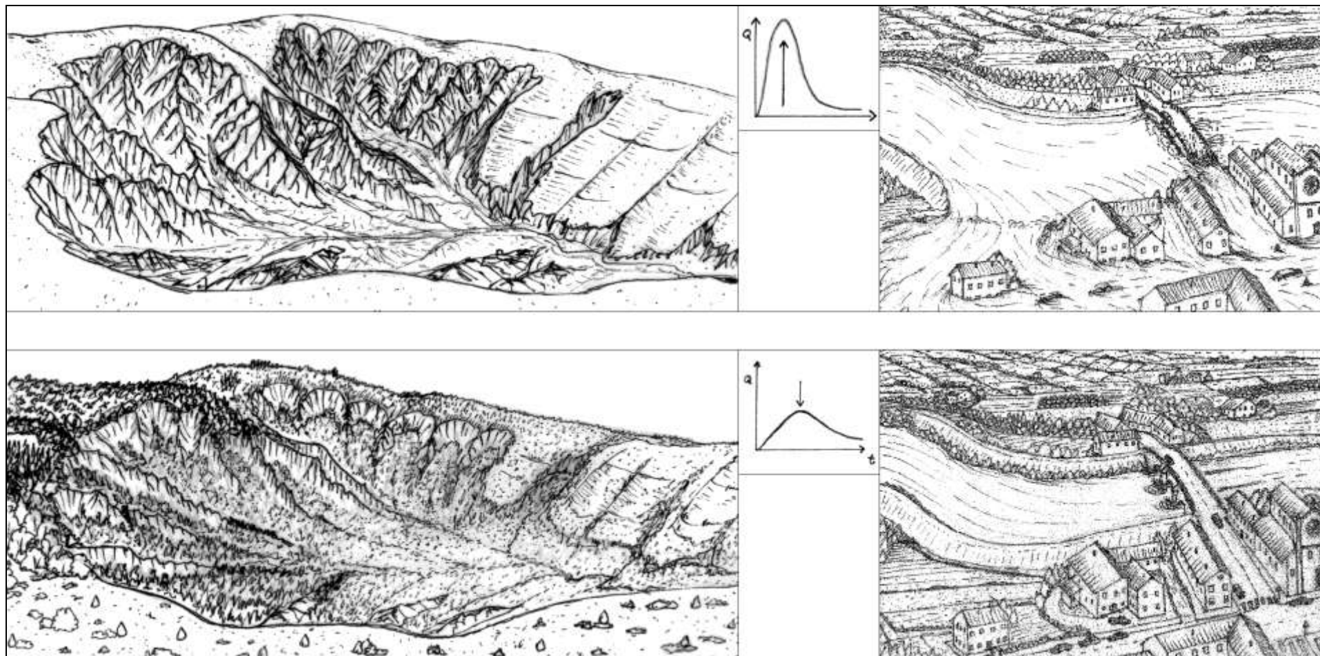
Figura 16 – Schema progettuale di massima dell'intervento di forestazione della piana inondabile.
