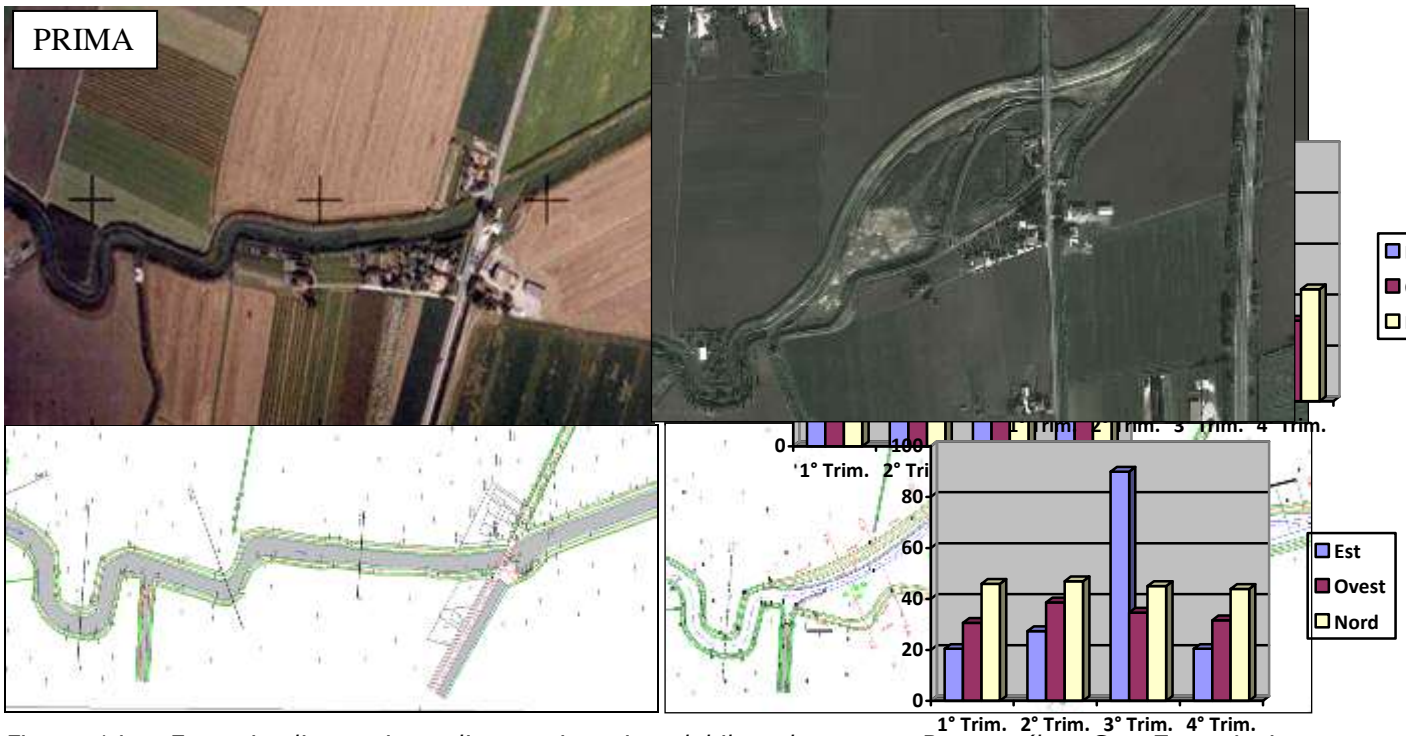
Figura 14 – Esempio di creazione di una piana inondabile sul torrente Bevano (loc. San Zaccaria in Comune di Ravenna)
