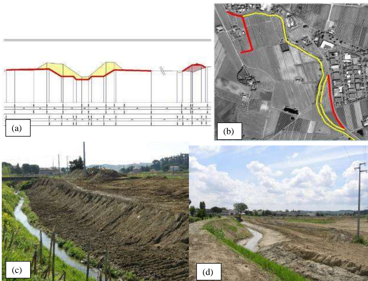
Figura 5 – Esempio di arretramento arginale sul torrente Pisciatello (Cesena). Un esempio simile al precedente, anche se con ampliamenti più contenuti, è quello relativo agli interventi per la mitigazione del rischio da esondazione sul torrente Pisciatello realizzato nel 2009-2010. Anche in questo caso in alcuni tratti è stata attuata la rimozione degli argini esistenti (in giallo in figura a e b) con parziale ricostruzione di un argine arretrato a protezione di elementi a rischio (in rosso in figura a e b), con conseguente incremento e diversificazione della sezione. In figura c e d si mostra il contestuale allargamento di sezione realizzato sul medesimo torrente. Intervento e foto: Servizio Tecnico di Bacino Romagna della Regione Emilia-Romagna.
