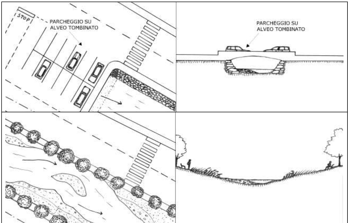
Figura 45 – Schema progettuale di massima dell'intervento. In alto a sinistra, nella visione planimetrica, è rappresentato un parcheggio realizzato tombinando un corso d'acqua, che torna a cielo aperto sulla destra del parcheggio (con direzione del flusso indicata dalla freccia). In alto a destra la medesima situazione vista in sezione, con il corso d'acqua coperto dal tombinamento. In basso è invece rappresentato in pianta (a sinistra) e in sezione (a destra) il medesimo sito dopo la rimozione del tombinamento e la riapertura del corso d'acqua. Disegni Regione Emilia-Romagna: Massimo Milandri.
