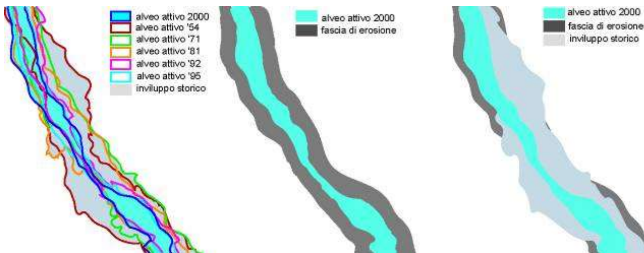
Figura 51 – Schema concettuale di massima dell'azione.
