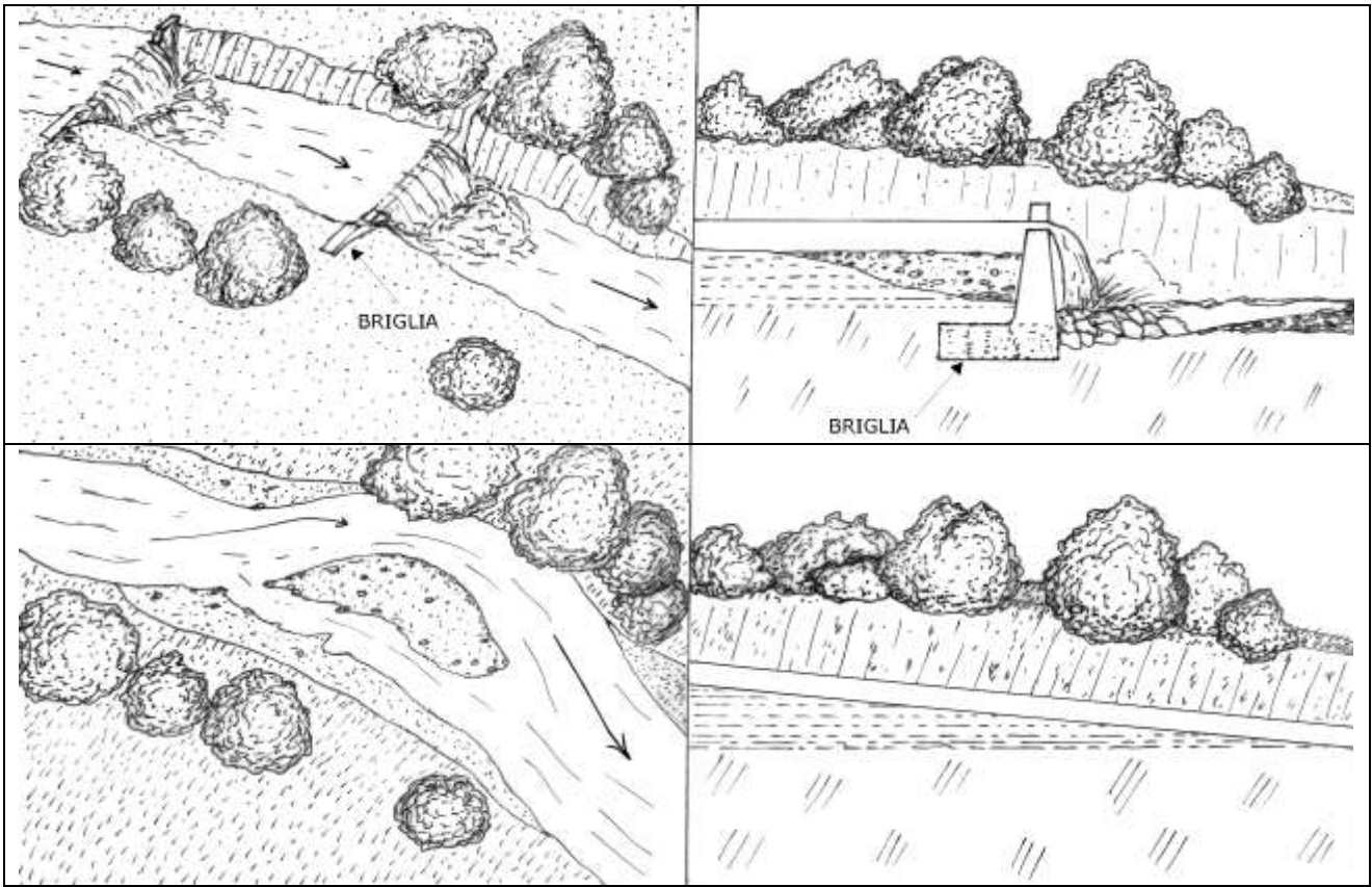
Figura 29 – Schema progettuale di massima dell'intervento. Disegni Regione Emilia-Romagna: Massimo Milandri.
