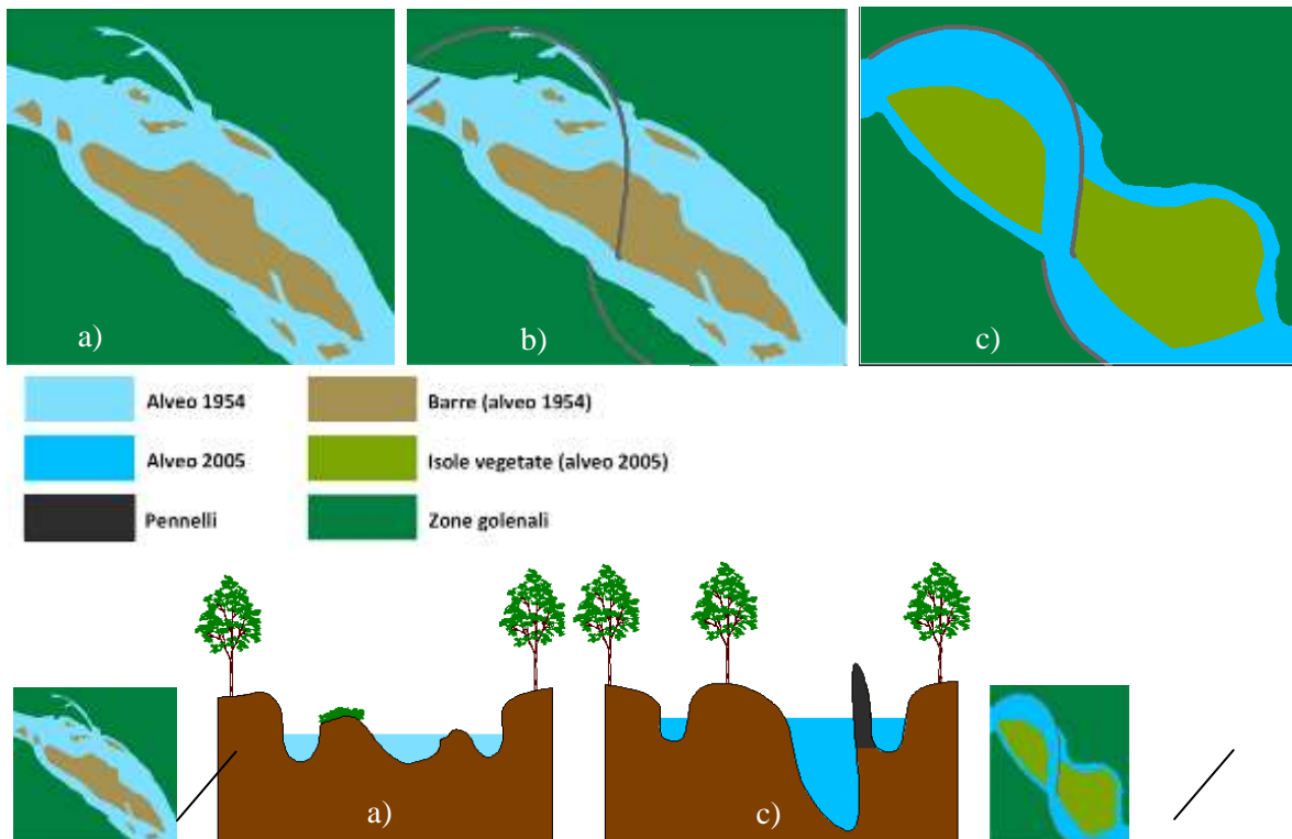
Figura 26 - A partire dagli anni cinquanta il tratto di fiume Po compreso tra Cremona e foce Mincio è stato progressivamente sistemato per la navigazione a corrente libera tramite l'impostazione del tracciato del canale di magra secondo una serie di curve e controcurve regolari. Fino al 1954 (a) l'alveo era caratterizzato da canali multipli e barre attive non vegetate. In seguito, a causa della costruzione dei pennelli (b) e soprattutto di un complessivo squilibrio del bilancio sedimentario indotto principalmente dalle escavazioni in alveo tra gli anni '60 e gli anni '80 e dalla costruzione dello sbarramento di Isola Serafini, il canale navigabile si è progressivamente inciso, diventando l'alveo principale del fiume, mentre gli altri canali hanno subito nella maggior parte un processo di interrimento. I canali a tergo dei pennelli hanno infatti funzionato come trappola per sedimenti, essendo inondati da valle e quindi con velocità molto basse che hanno favorito il deposito del trasporto in sospensione. Parallelamente, nel corso degli anni, le barre si sono progressivamente consolidate e vegetate, diventando isole stabili la cui quota è attualmente paragonabile a quella della piana inondabile circostante. L'assetto attuale (c, figure riferite al 2005) è caratterizzato da un alveo principale che si appoggia ai pennelli longitudinali e canali secondari poco profondi e disconnessi a monte per la maggior parte delle portate in alveo. Coerentemente con il Programma generale di Gestione dei Sedimenti dell'Autorità di bacino del Fiume Po e puntando a invertire il processo di semplificazione e banalizzazione dell'ambiente fluviale in corso, pur garantendo la navigabilità a corrente libera, AIPO (Agenzia Interregionale per il fiume Po) ha avviato interventi con lo scopo di ripristinare e mantenere rami laterali ancora parzialmente attivi, migliorando l'assetto morfologico ed ecologico del fiume, e di recuperare almeno in parte la continuità laterale del trasporto solido mediante la riattivazione di processi erosivi ordinari in corrispondenza dei sedimenti alluvionali presenti a tergo dei pennelli. Gli interventi sono stati progettati in modo da abbassare i pennelli alla quota del profilo per una portata pari a 800 m 3 /s, garantendo una connessione idraulica molto più frequente rispetto all'attuale. In diversi casi gli interventi hanno anche l'obiettivo di ridurre, grazie alla ripartizione della portata nei rami laterali, le sollecitazioni in corso di piena sul fondo alveo e sulla sponda opposta rispetto al
