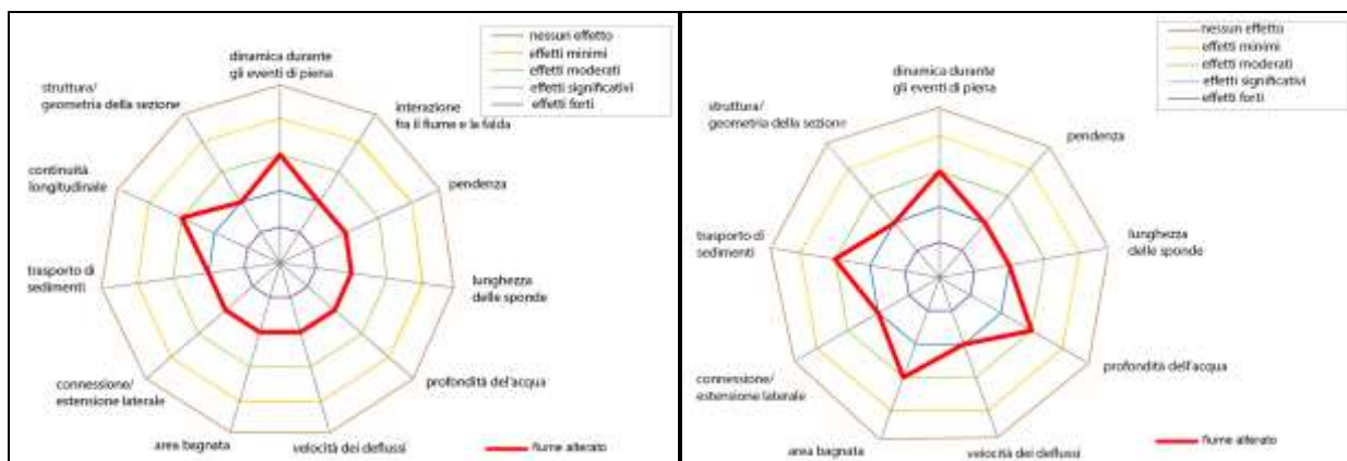
Figura 54 – Rappresentazione dell'intensità degli impatti indotti dalla realizzazione di arginature (grafico a sinistra) e di interventi di rettificazione (a destra) su una serie di indicatori idromorfologici. Per le arginature si nota un'interferenza molto significativa (linea rossa) per tutti gli indicatori ad esclusione della "continuità longitudinale" e della "dinamica durante gli eventi di piena" (moderate). Per le rettificazioni i maggiori impatti (linea rossa) si hanno su "struttura geometrica della sezione", "pendenza", "lunghezza delle sponde", "connessione/estensione laterale" e "velocità dei deflussi" (da Alonso C. et al., 2011, modificata).
