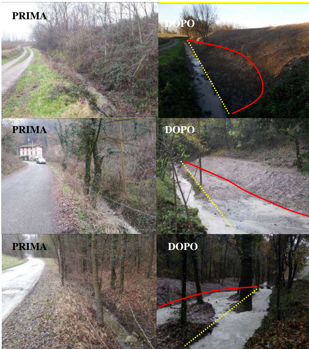
Figura 10 - Esempio di creazione di piana inondabile in un corso d'acqua non arginato mediante abbassamento del piano campagna (rio Enzola, Provincia di Reggio Emilia).
