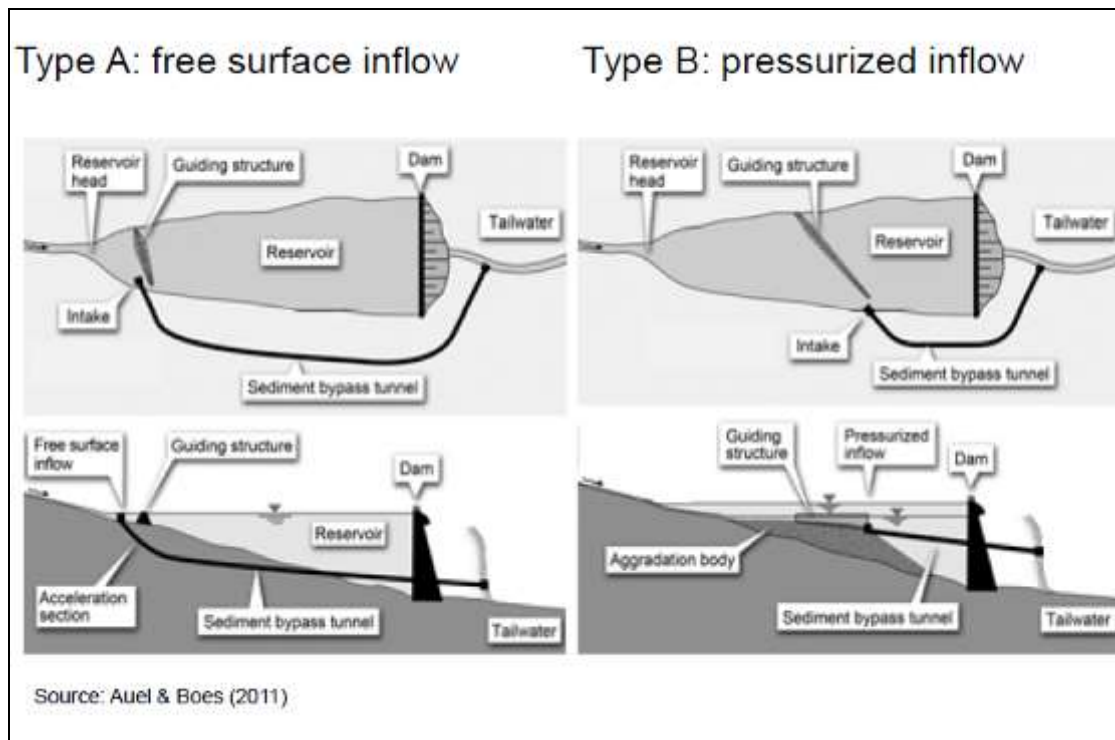
Figura 36 – Costruzione di un by-pass per il transito dei sedimenti grossolani a valle di una diga (Fonte: Auel, C. & Boes, R.M. (2011).
