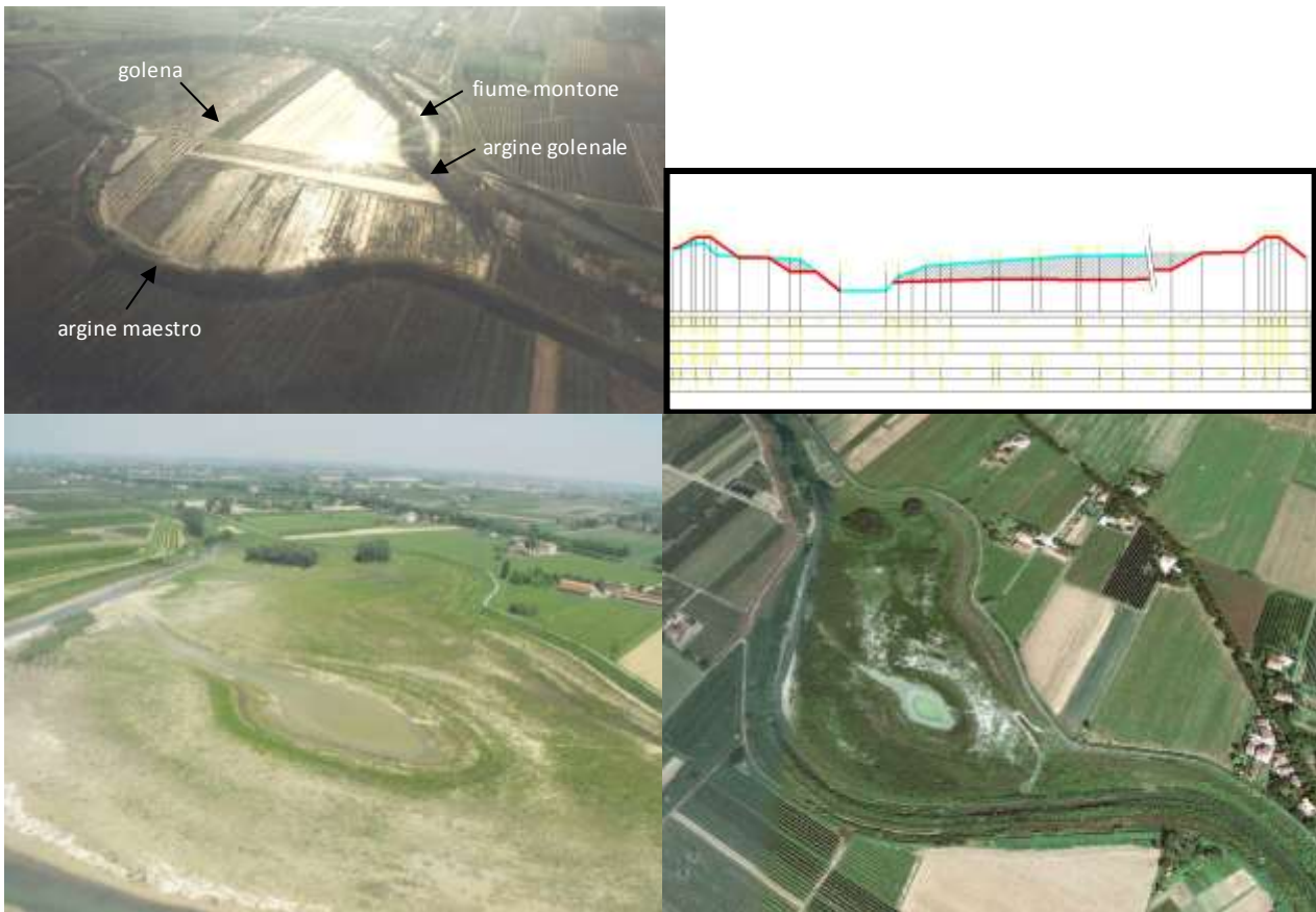
Figura 13 – Esempio di creazione di piana inondabile in un fiume arginato mediante abbassamento del piano campagna di una golena presente lungo il fiume Montone (Forlì).
