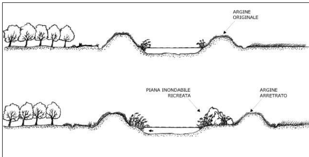
Figura 2 – Schemi progettuali di massima dell'intervento. In entrambi i casi si prevede la rimozione con ricostruzione arretrata dell'argine originariamente in frodo. Disegno Regione Emilia-Romagna: Massimo Milandri.
