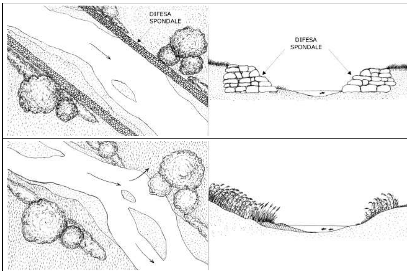
Figura 20 - Schema progettuale di massima dell'intervento. Disegni Regione Emilia-Romagna: Massimo Milandri
