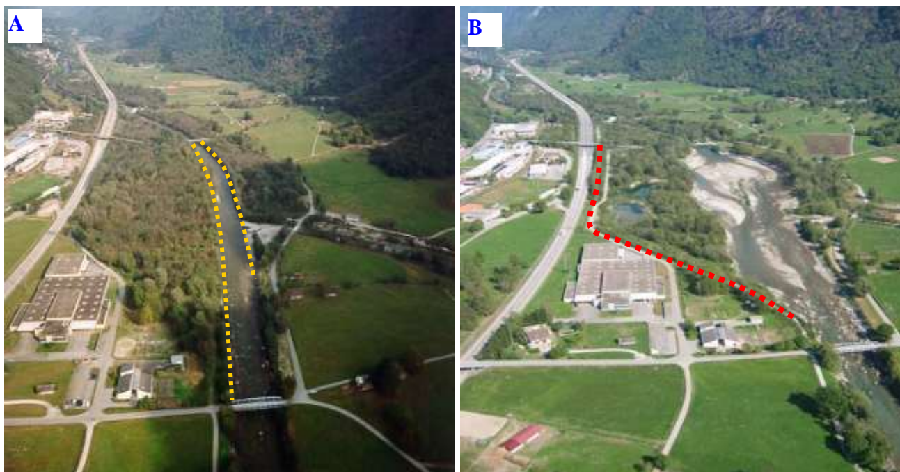
Figura 21 – Esempio di rimozione di difese spondali e rivitalizzazione della zona golenale Pascoletto sul Torrente Moesa (Svizzera).
