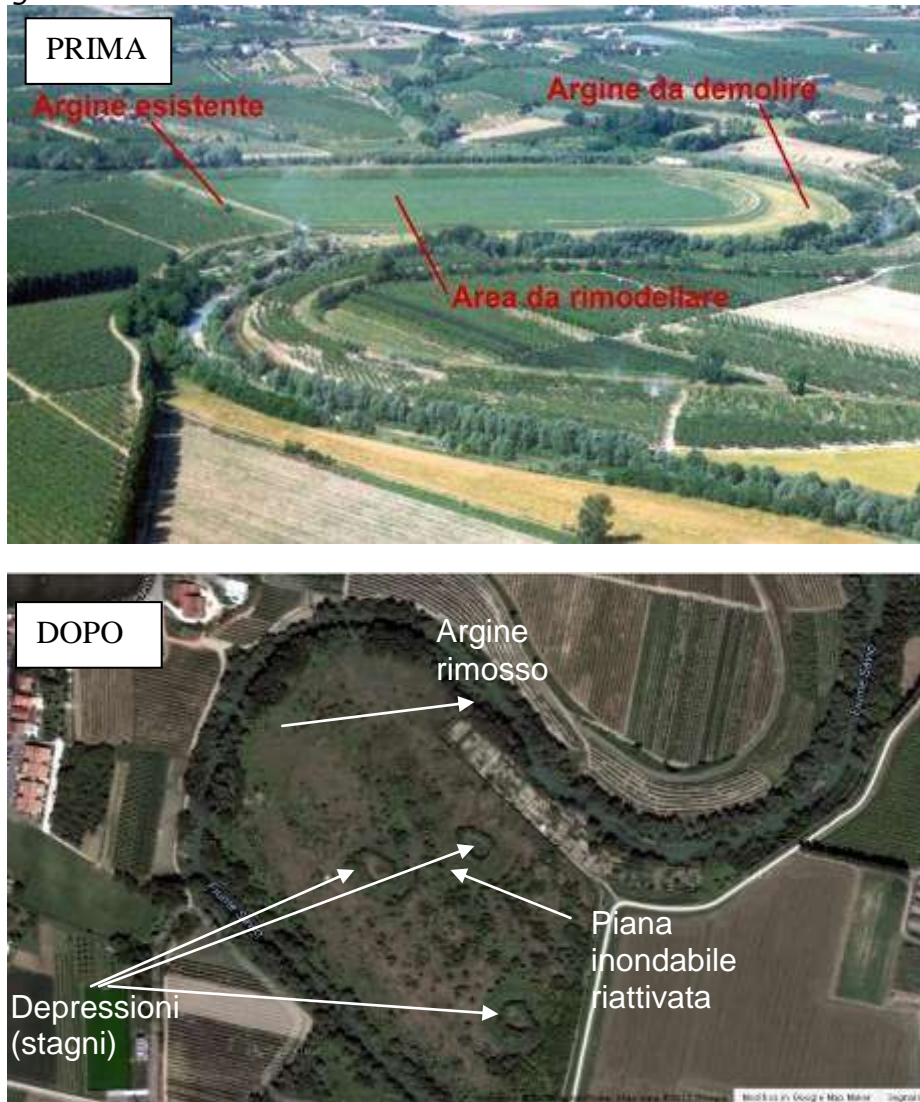
Figura 4 – Esempio di eliminazione di un argine sul fiume Savio nei pressi di Cesena. L'intervento è consistito nella demolizione di un argine interno ad un meandro e nella rimodellazione, tramite abbassamento e creazione di depressioni, di una vasta area di decantazione di sedimenti di un ex-zuccherificio ai fini di ricostituire un'area alluvionabile frequentemente allagabile. L'intervento, oltre a migliorare l'andamento complessivo del fiume Savio sotto il profilo idraulico, ha permesso la realizzazione, con una adeguata piantagione di essenze arboree idonee (circa 6.000 piante), di una zona naturalistica di notevole interesse ambientale. Inoltre sono state realizzate all'interno dell'ansa alcune depressioni umide protette (tre piccoli stagni), per favorire l'insediamento di specie faunistiche e l'aumento della biodiversità ambientale. Intervento e foto: Servizio Tecnico di Bacino Romagna della Regione Emilia-Romagna.
