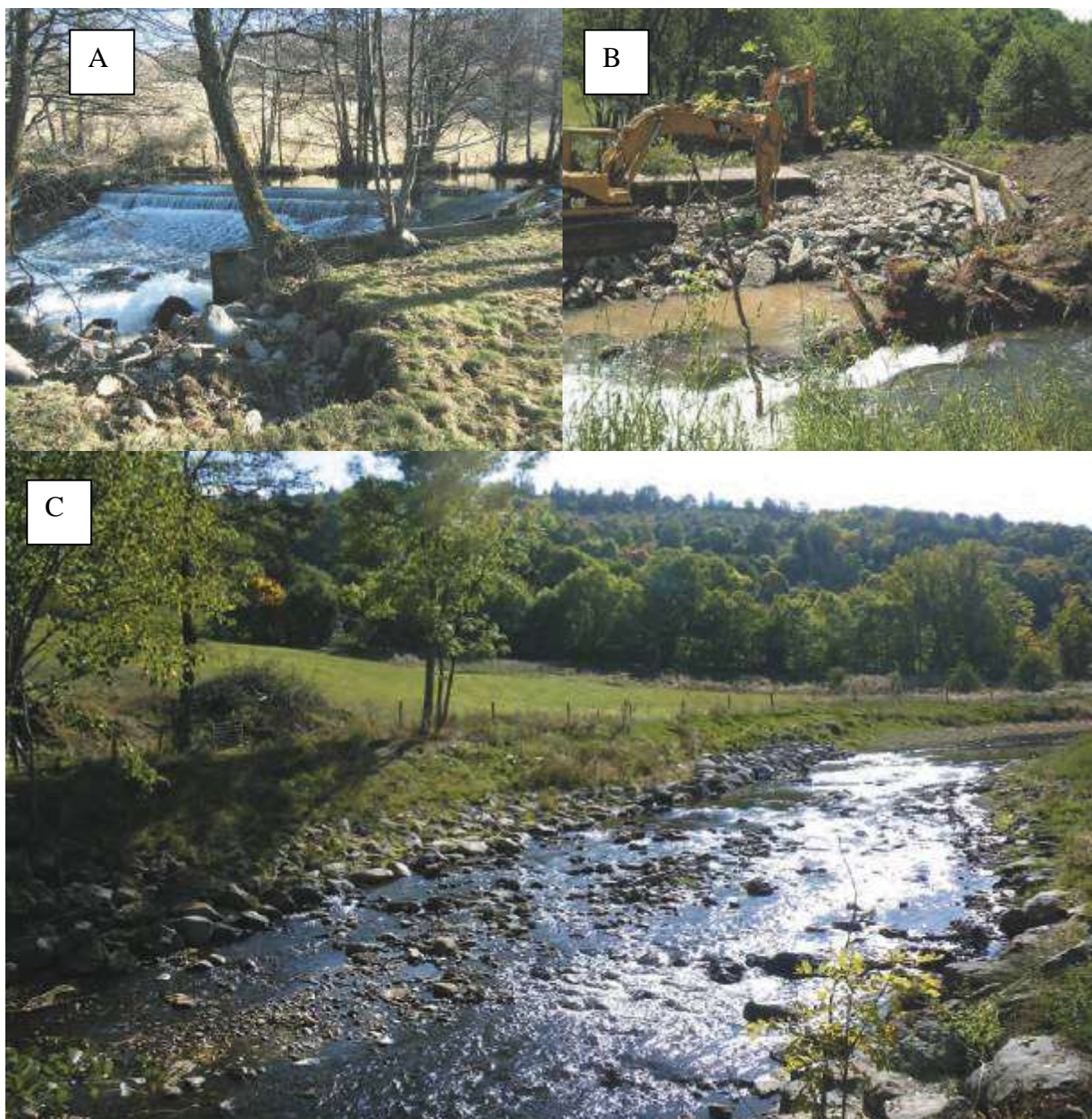
Figura 30 – Rimozione di una briglia (visibile in A) sul torrente Alagnon, un affluente dell'Allier nel bacino della Loira (Francia).
