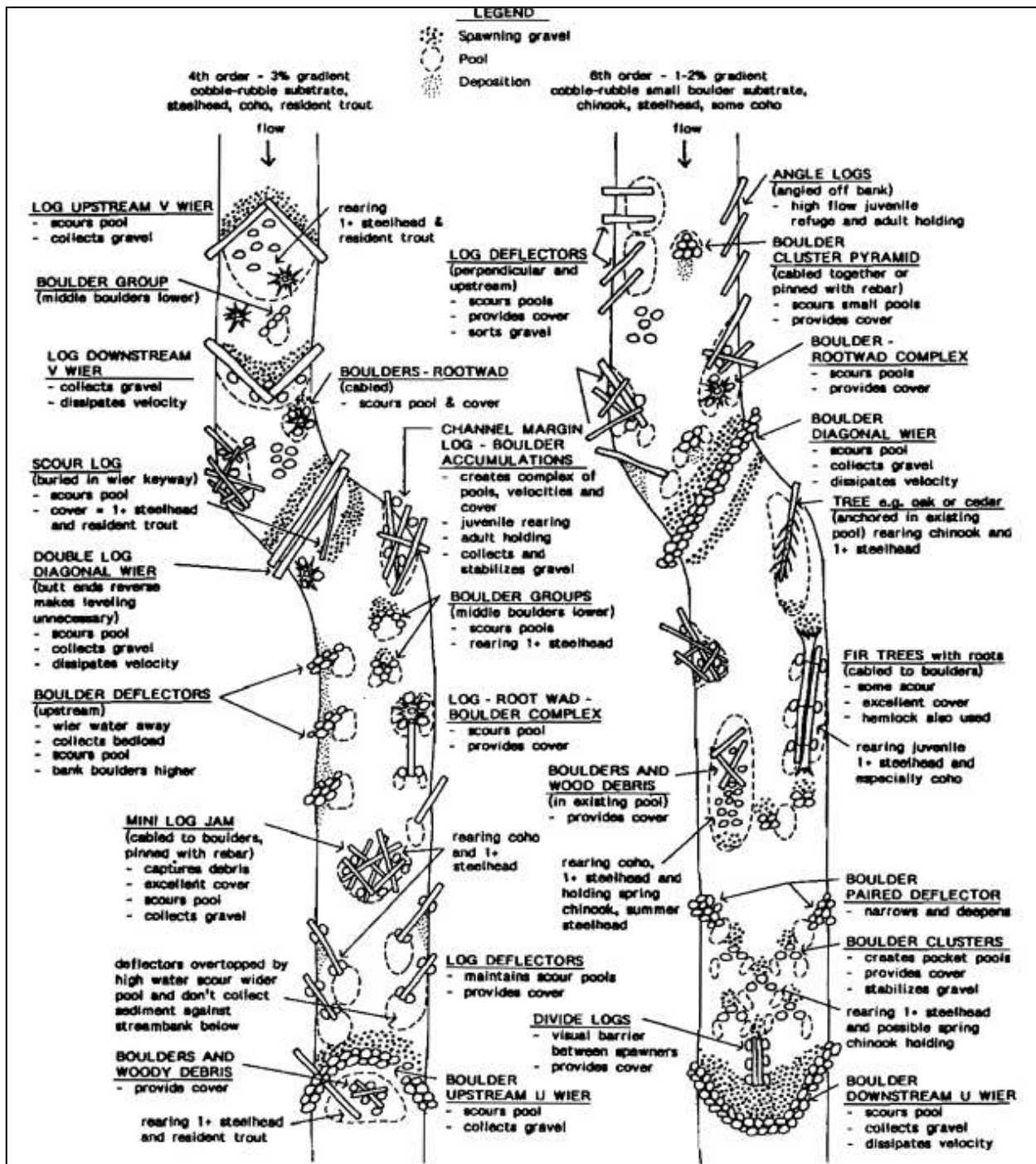
Figura 18 – Possibili tipologie di intervento per l'incremento della scabrezza e la creazione di habitat in alveo. (Fonte: Ministry of environment, lands and parks – British Columbia, 1997)
