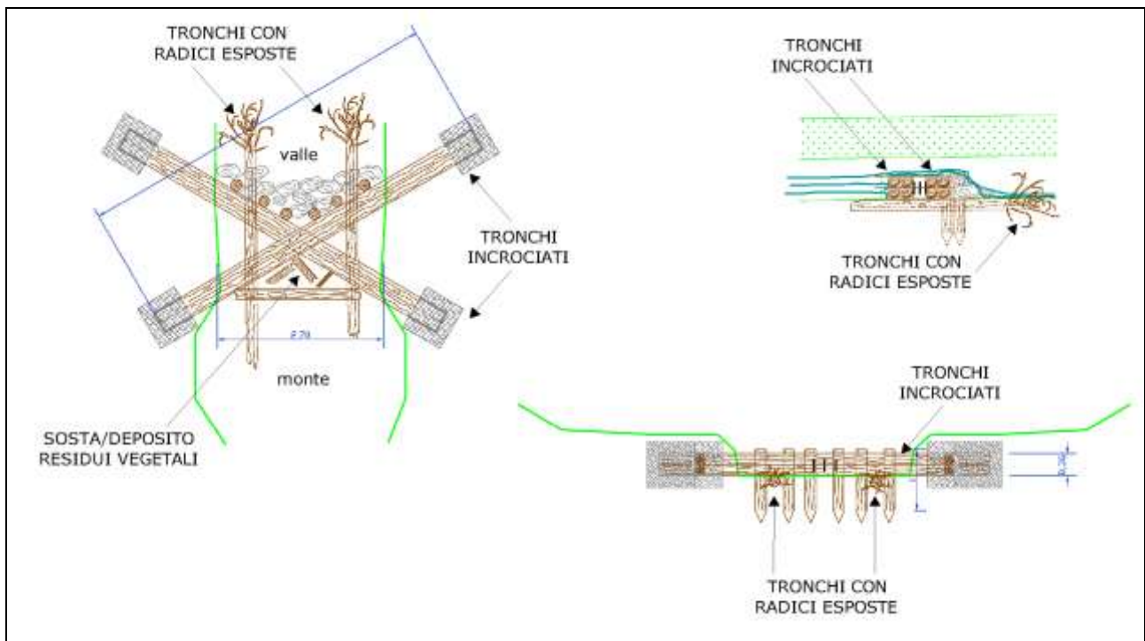
Figura 37 - Schema progettuale di massima dell'intervento di costruzione di strutture trasversali atte ad aumentare la capacità di sedimentazione e rialzare il livello dell'alveo Immagine: Consorzio di Bonifica dell'Emilia Centrale (RE).
