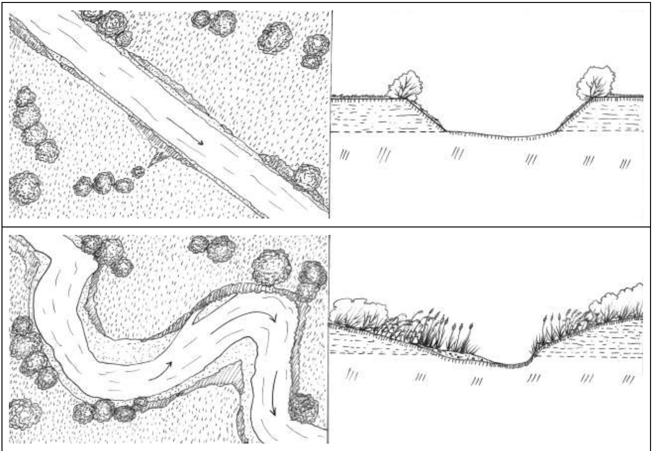
Figura 49 – Schema progettuale di massima dell'intervento Disegni Regione Emilia-Romagna: Massimo Milandri.
