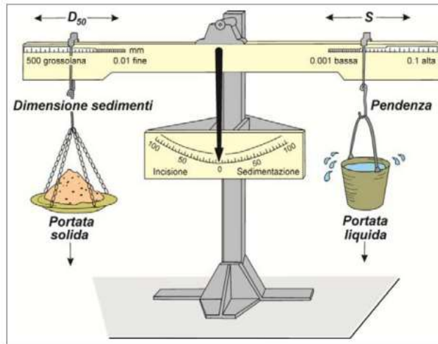
Figura 1 - Modello concettuale delle risposte di un alveo fluviale ad alterazioni dell'equilibrio dinamico, tratto da Manuale IDRAIM di ISPRA - Istituto Superiore per la Protezione e la Ricerca Ambientale (2014)
